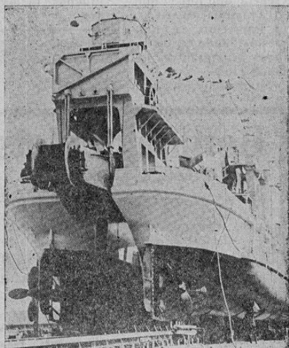
La «Pas de Calais II», la más poderosa draga que jamás se ha construido, al ser botada al agua en Dunkirk, Francia, para ser utilizada en el dragado del puerto de Boulogne-sur-Mer. Posee 49 palas que pueden dragar a una profundidad de 23 metros, y a una velocidad de 15 paladas por minuto.
